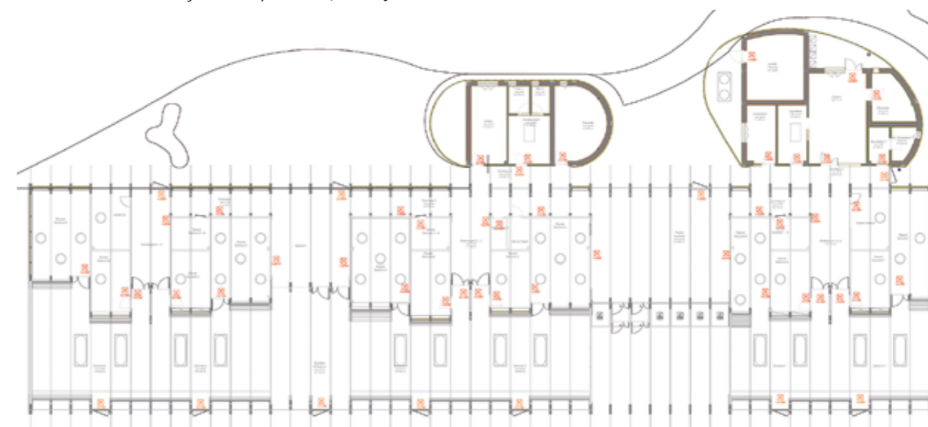
LA DISPOSIZIONE in planimetria delle lampade dell'impianto di illuminazione di emergenza.
